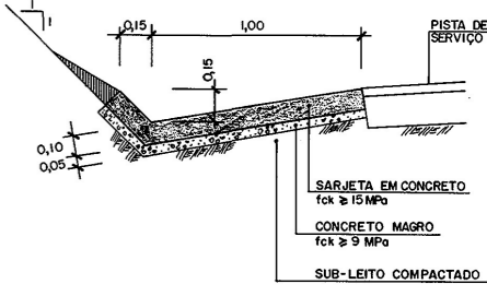
DETALHE DA SARJETA ESC. 1:20
